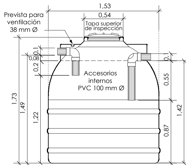
SECCIÓN TRANSVERSAL
